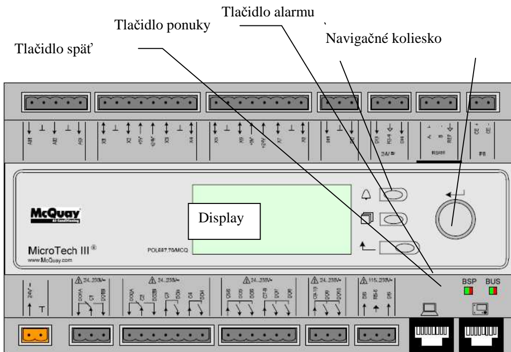
Obrázok 1, ovládač jednotky
