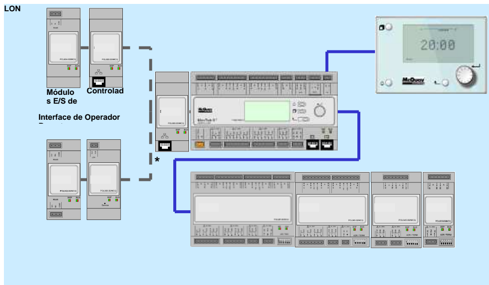
Figura 6, estrutura de hardware
