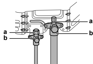
a Servisná prípojka b Uzatvárací ventil
