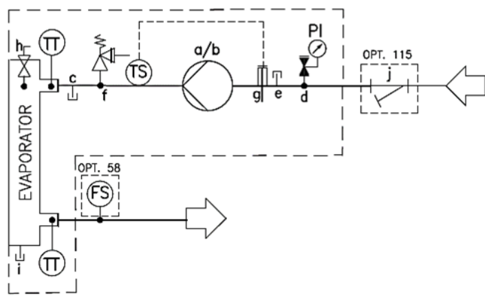
Slika 7 - Vezava vodovodnih cevi za izparilnik (opt.78-79-80-81)
