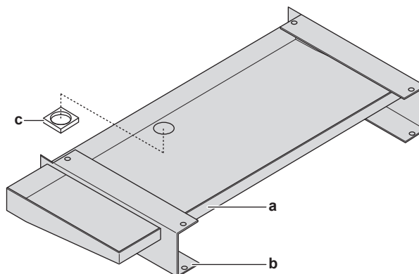
a Odtoková vaňa b Nosíky tvaru U
