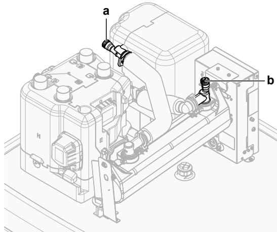
a, b Manuálny odvzdušňovací ventil
