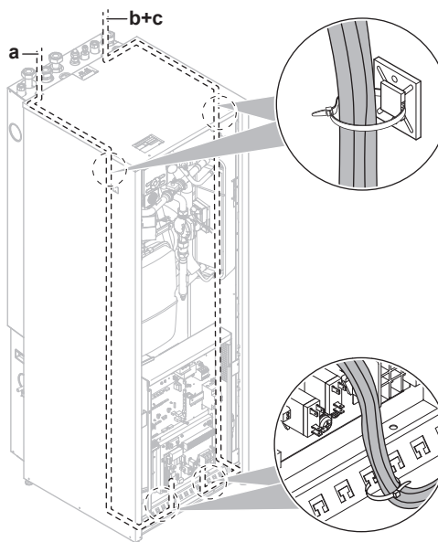
4 Kábel upevnite pomocou káblových spôn, aby sa zaručilo uvoľnenie napätia. Kábel sa NESMIE dostať do kontaktu s potrubím a ostrými hranami.
