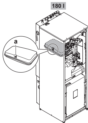
a Schraderov ventil
