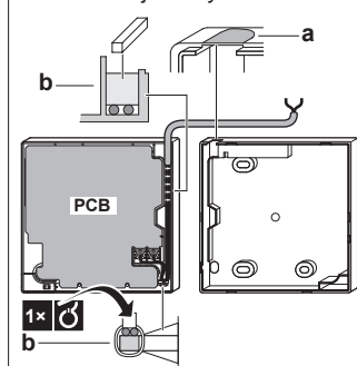
4C Z vrchnej strany
