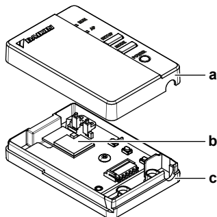
a Horný kryt b Doska s tlačnými obvodymi bezdrôtového adaptéra LAN c Spodný kryt
