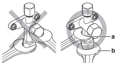
a Kľúč na maticu b Momentový kľúč
